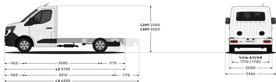
sasiu cabina (mm)
